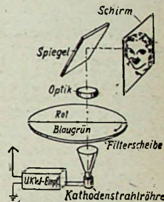
Abb. 5. Fernsehempfang mit zweiteiligem Farbfilter.
