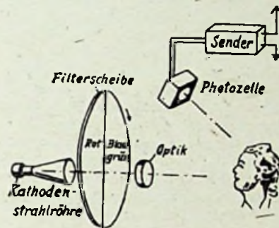
Abb. 4. Zweifarbiges Fernsehensendung (Baird 1941).
