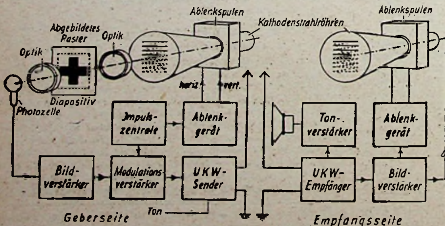
Schema einer Schwarz-Weiß-Fernsehübertragung mit Leuchtschirmabtaster auf der Geberseite Zeichnung: Trester
