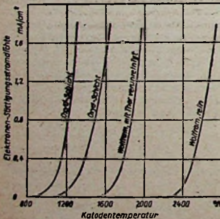
Emissionskennlinien einiger wichtiger Kathodenbaustoffe Zeichnung: Trester
