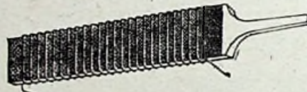
Abb. 2. Beispiel der Anwendung einer hochfrequenten Induktionsheizung zur Oberflächenhärtung von Feilen (Schematische Darstellung)
