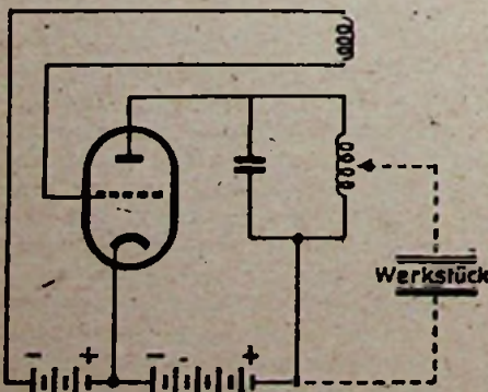
Abb. 4. Grundständliches Schaltbild eines Röhrenoszillators für Dielctrikheizung mittels Kondensatorwärme
