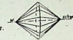
Abb. 2c. Farbdreieck.
